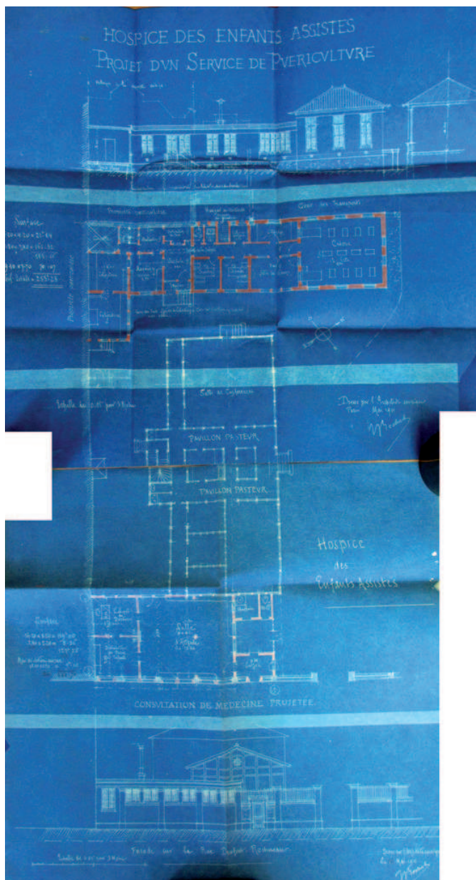
1911- JUSTIN-JEAN-MARIE ROCHET, ARCHITECTE. Hospice des enfants assistés : plans et élévation de l'institut de puériculture du docteur Gastion Variot. Archives de l'Assistance publique des hôpitaux de Paris, Catalogue Fosseyeux, 791 Foss-36/2.
