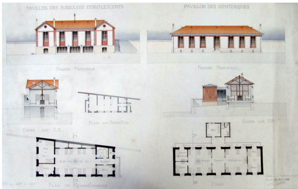
1886 - PAUL-MARIE GALLOIS, ARCHITECTE. Hospice des enfants assistés : les pavillons des rubéoleux convalescents et des diphtériques, plans et élévations. Archives de l'Assistance publique des hôpitaux de Paris, Plans, 793 Foss-27.
